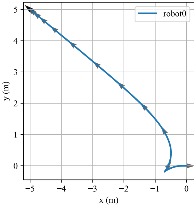
Trayectoria del robot
